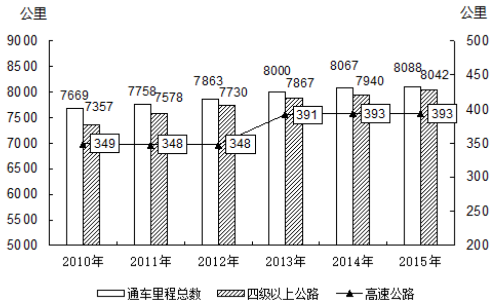
图7 2010-2015年全市公路通车里程
