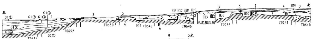
图五// T0640—T0654东壁剖面图
