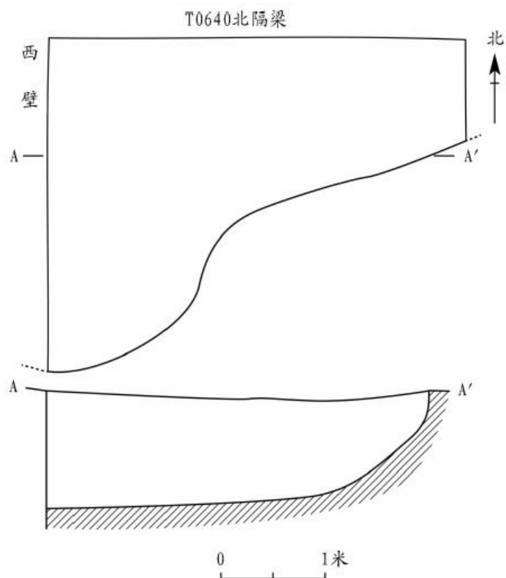
图八// H29平、剖面图
