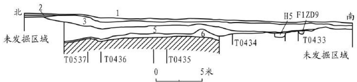
图四// T0433—T0436东壁、T0537西壁剖面图
