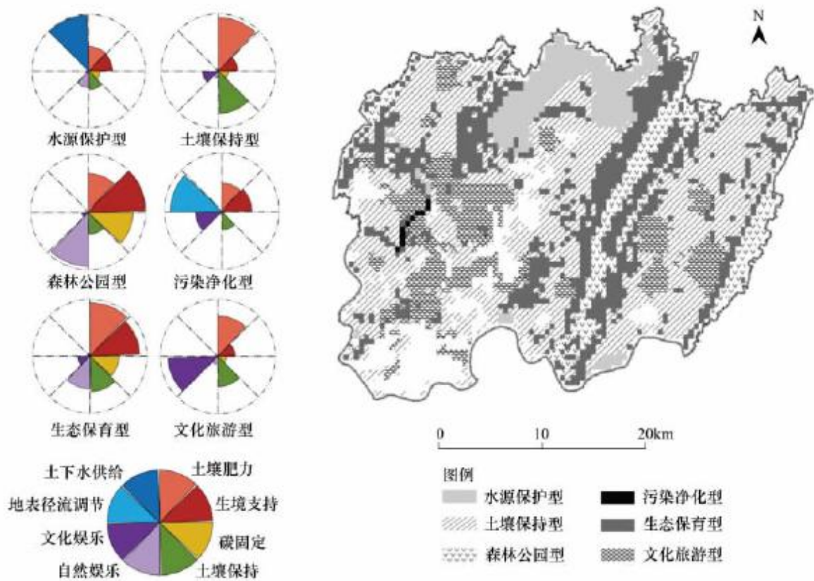
图 2 2010 年重庆两江新区生态系统服务簇空间分布及簇模式图 Fig.2 Spatial distribution and patterns of ecosystem service bundle in Liangjiang, 2010
