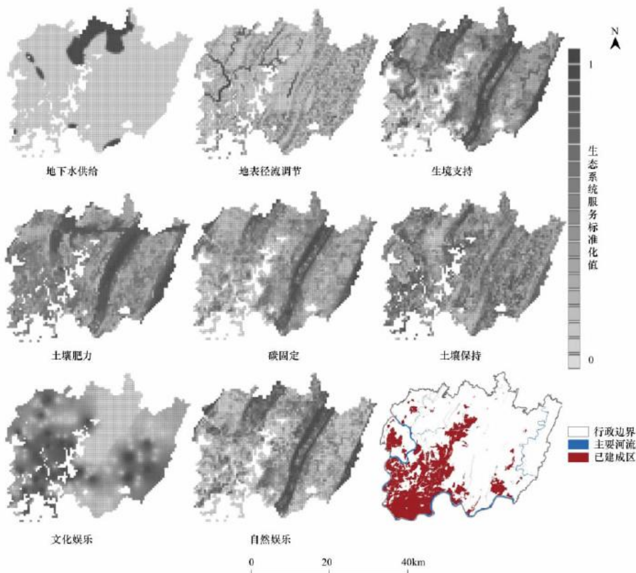
图1 2010年重庆两江新区生态系统服务空间分布图
