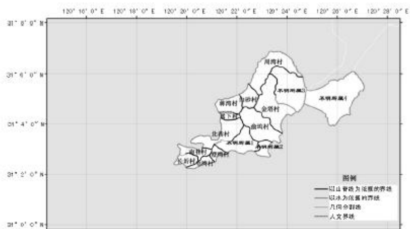
图 10 1529 年苏州府吴县东山村级行政区推断界线图
