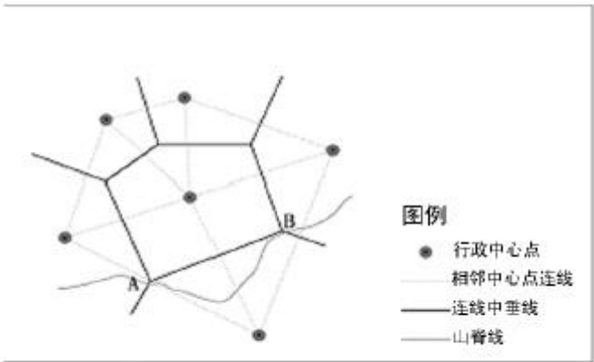
图 3 自然边界确定法示意图
