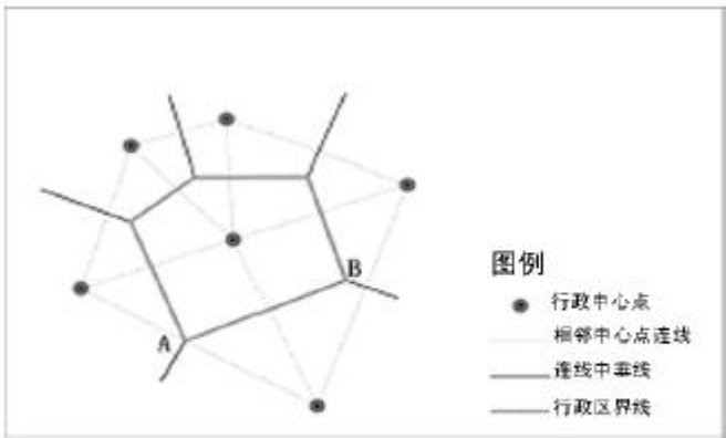
图1 几何边界确定法示意图
