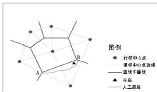
图 6 线状人文景观边界确定法示意图
