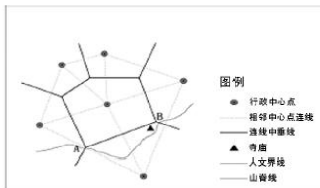
图 5 点状人文景观边界确定法示意图
