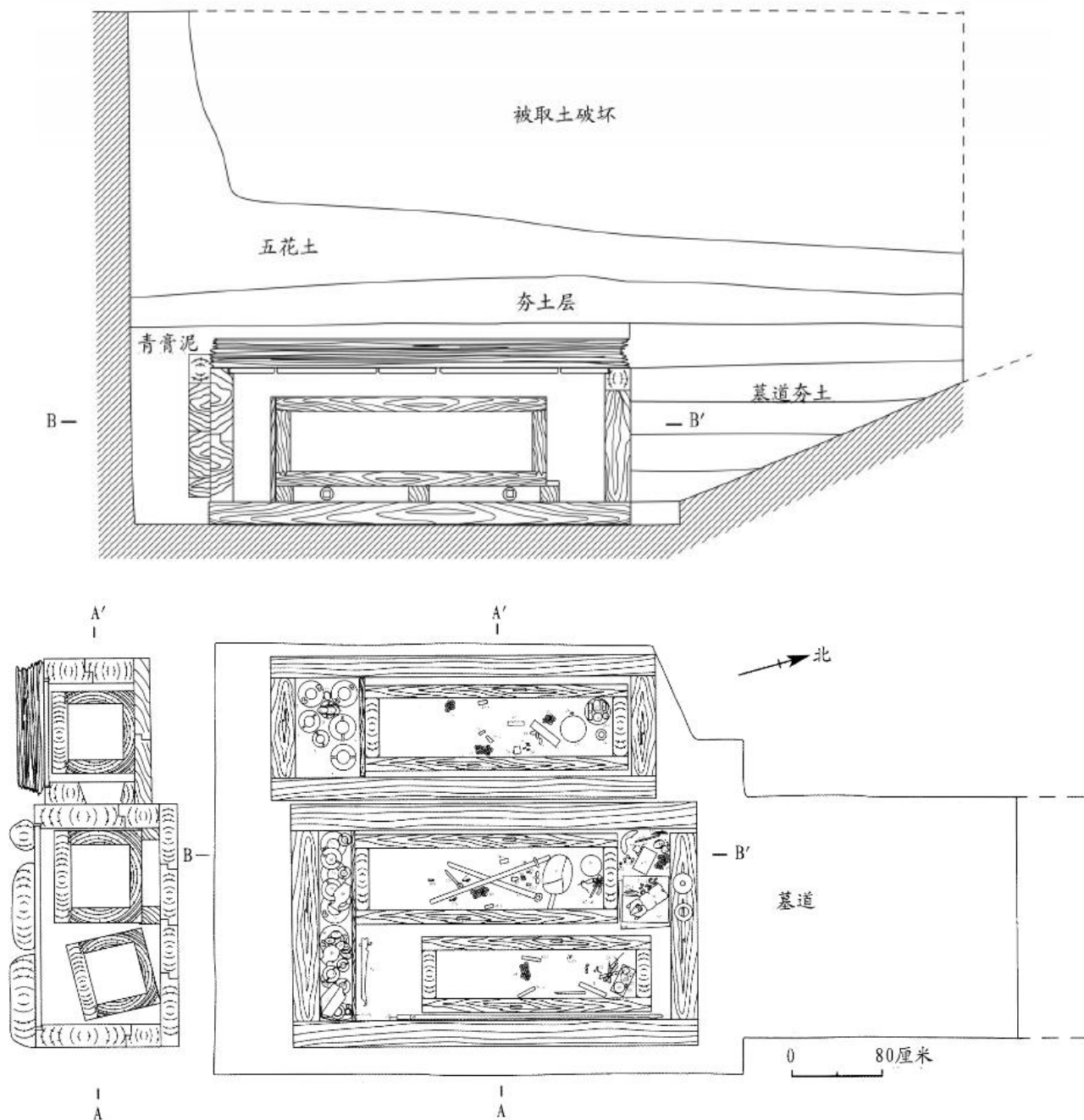
图二// M12平、剖面图
