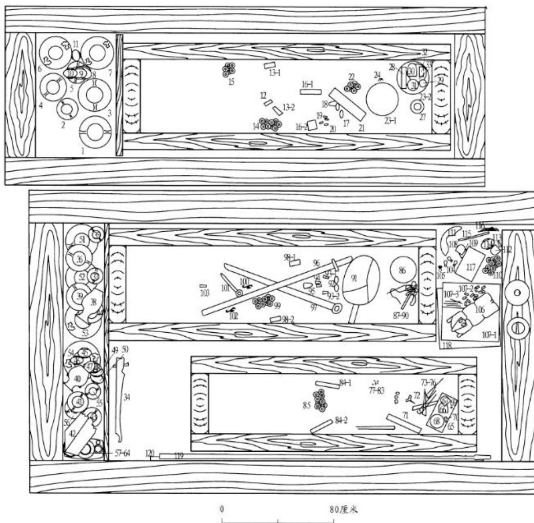
图三// M12出土器物分布图
