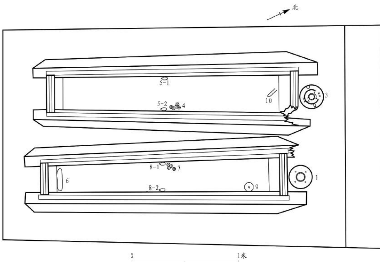
图三// M1平面图
