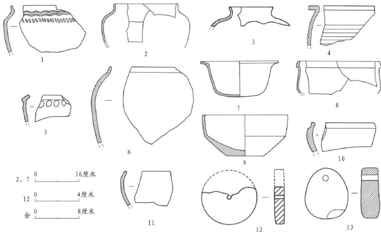
图一四// 陶罐、瓮、釜、钵、权形器、纺轮
