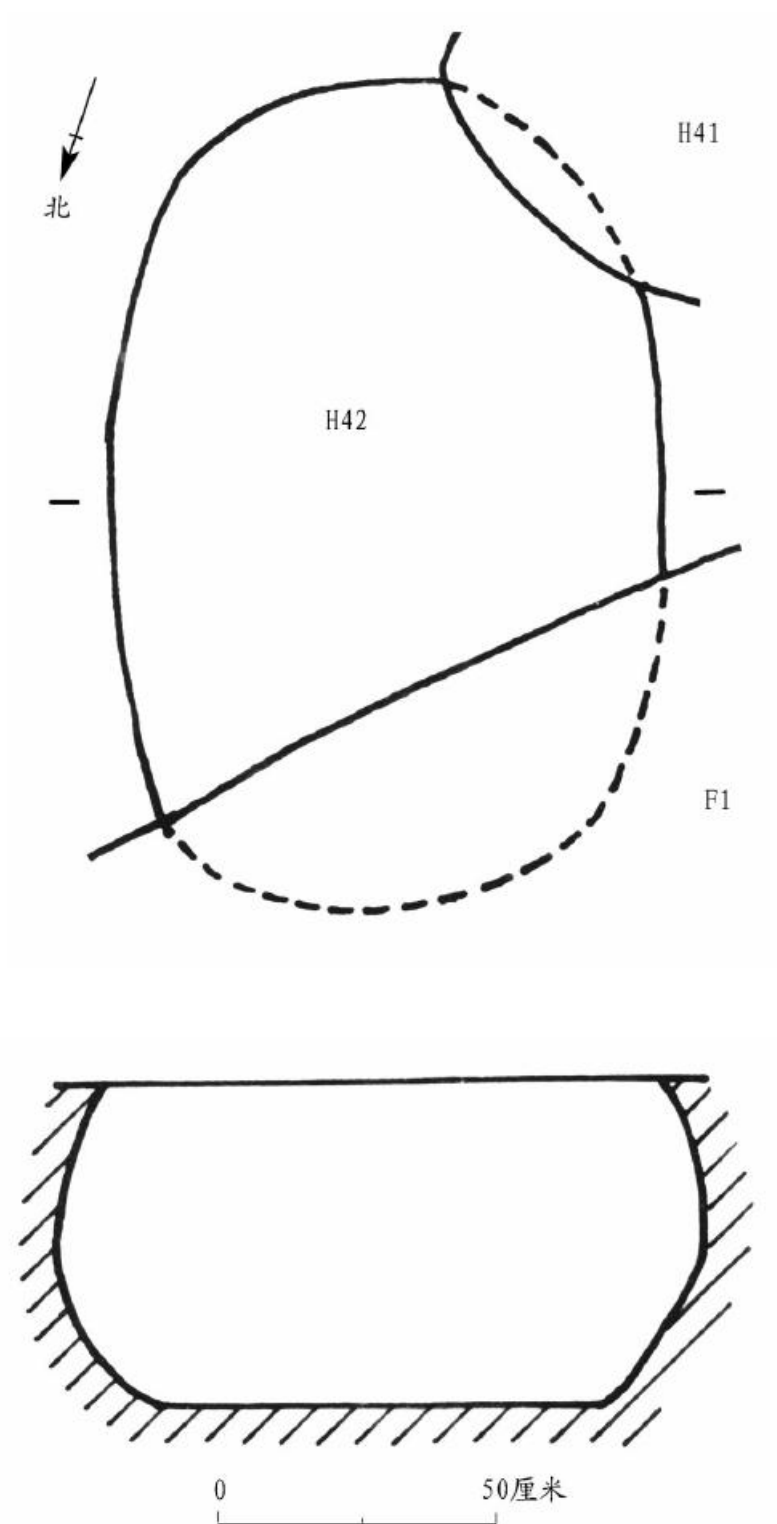
图一二// H42平、剖面图
