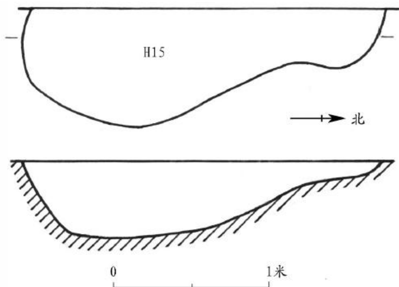
图二〇// H15 平、剖面图
