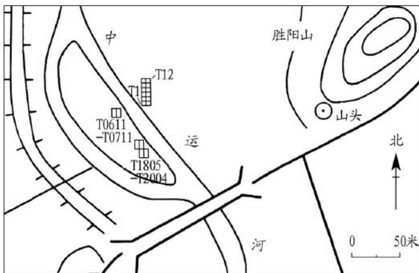
图二// 山头遗址探方分布图
