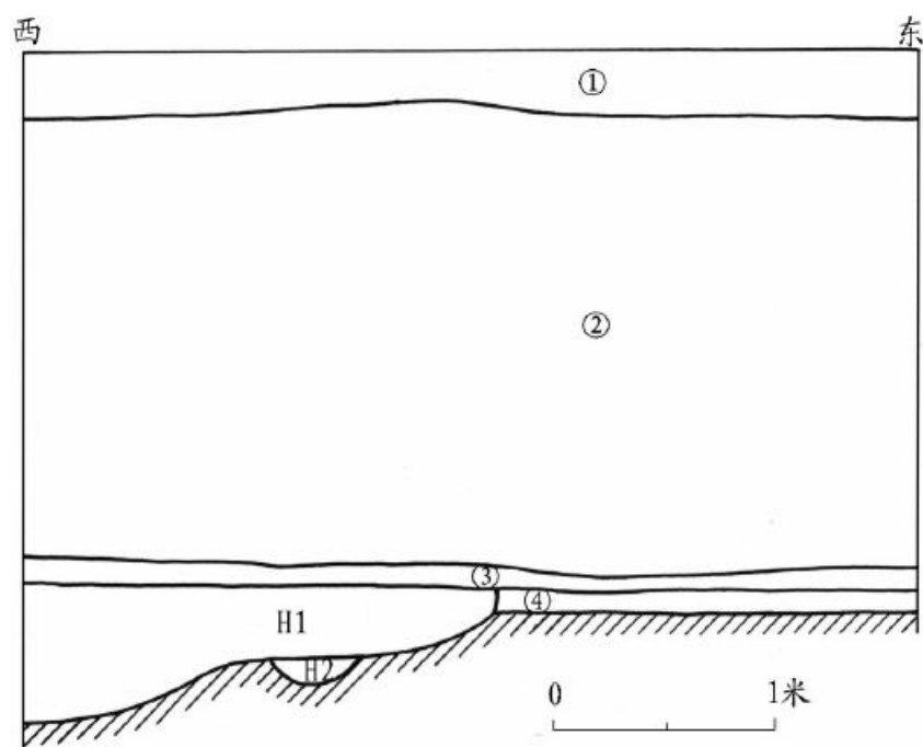
图六// T0711 北壁剖面图
