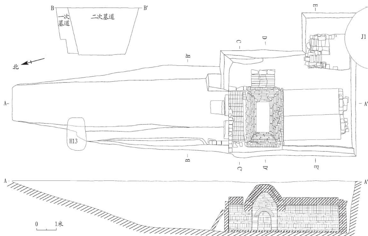
图三// M1平、剖面图
