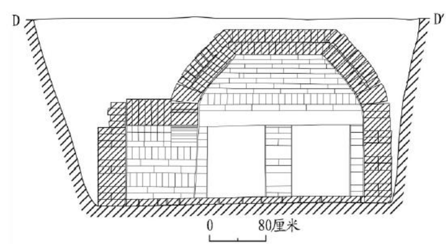
图八// M1前室横剖面图
