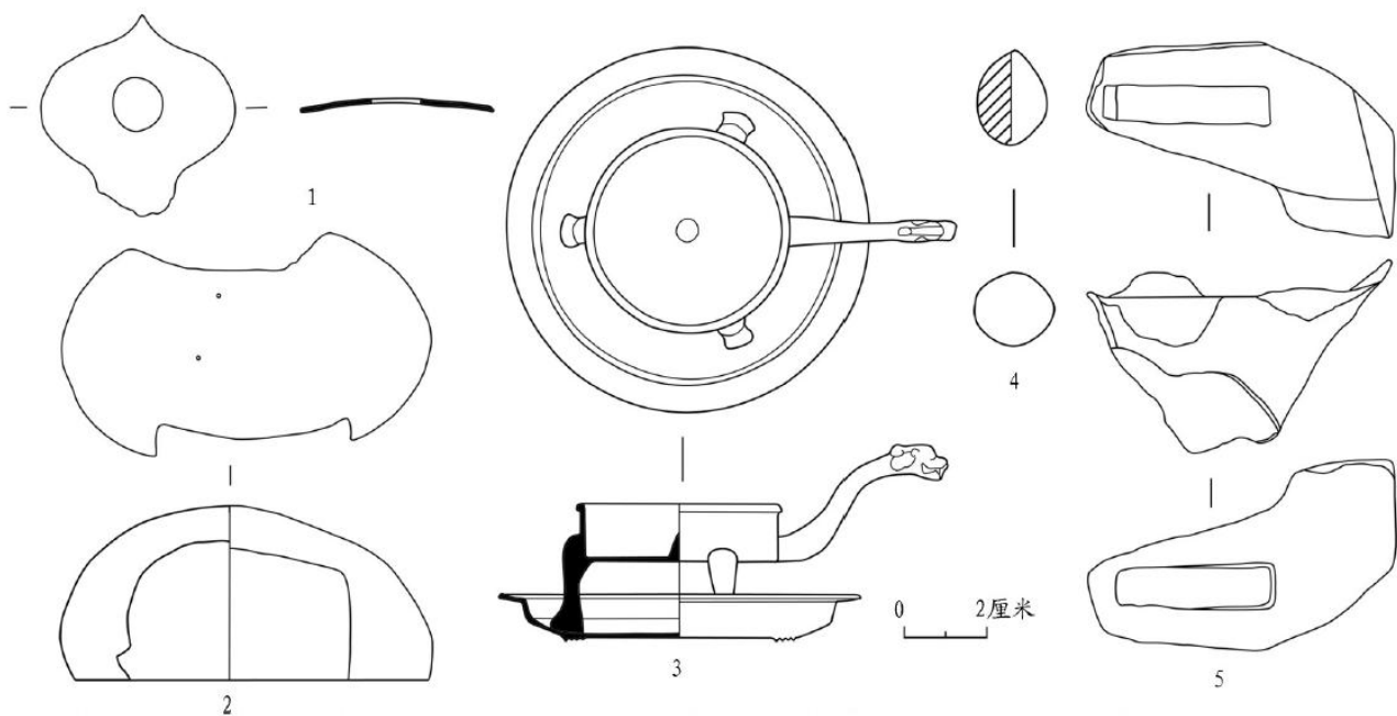
图一三// M1甬道出土器物
