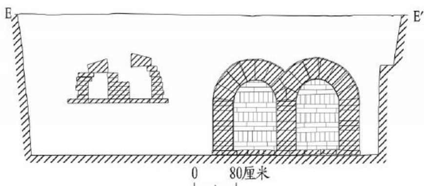
图一〇// M1后室横剖面图
