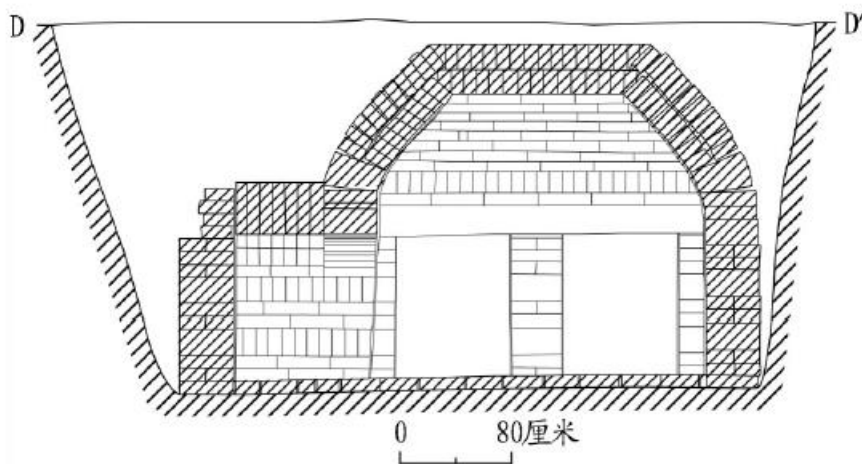
图八// M1 前室横剖面图
