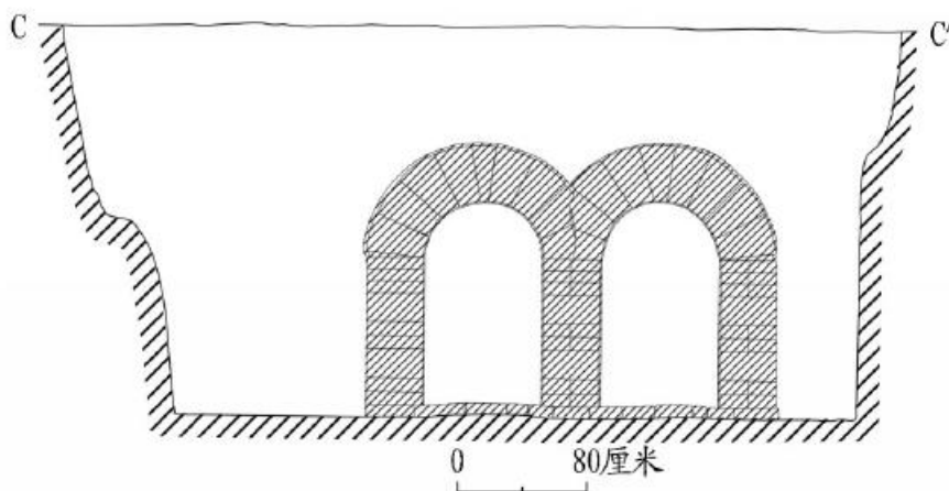
图七// M1 甬道横剖面图
