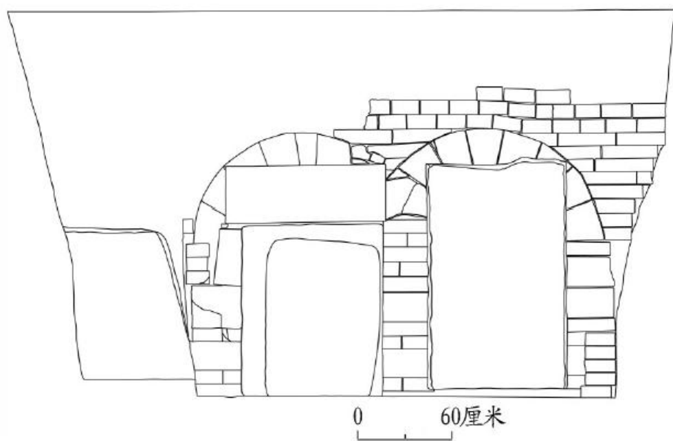
图六// M1 封门正视图
