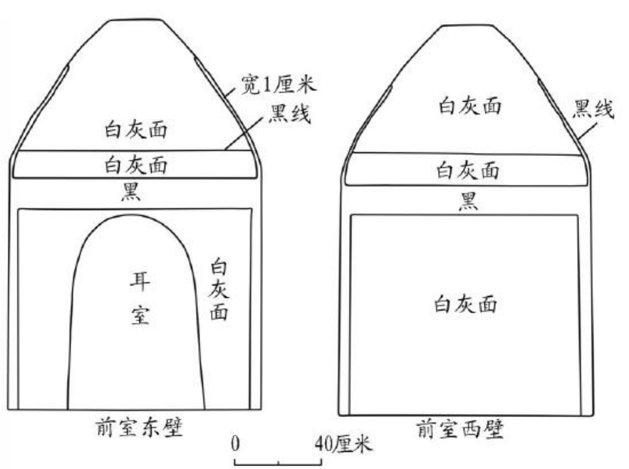
图九// M1前室影作正视图
