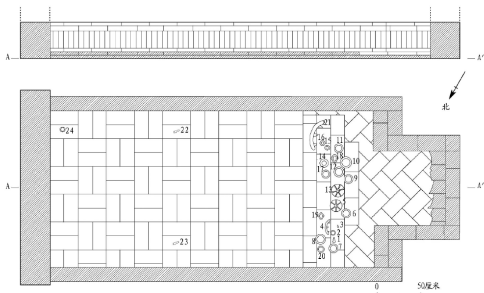
图二// YM1 平、剖面图
