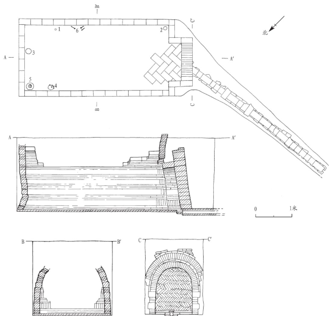
图三// M1平、剖面图
