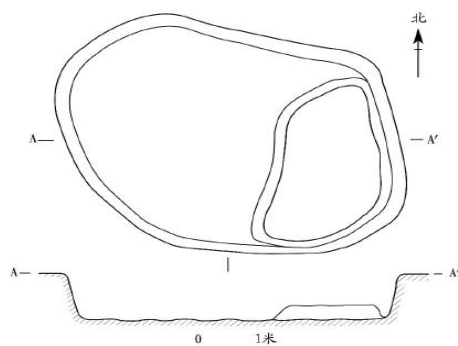
图八// H15平、剖面图
