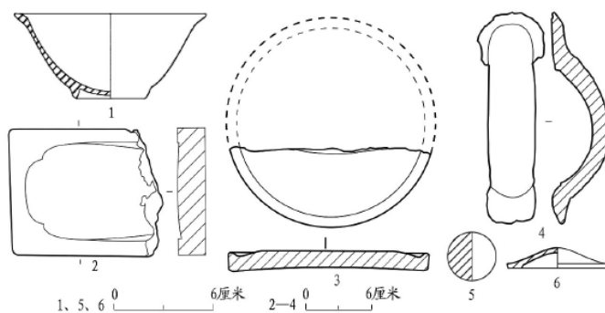
图一三// 出土陶器 1.碗(H4:5) 2、3.碗(H4:1、T0202⑤:2) 4.把手(T0204④:6) 5.球(H12:1) 6.器盖(H15:14)
