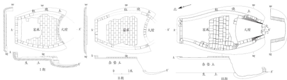
图六// Y2各期平、剖面图 1. I期 2. II期 3. III期
