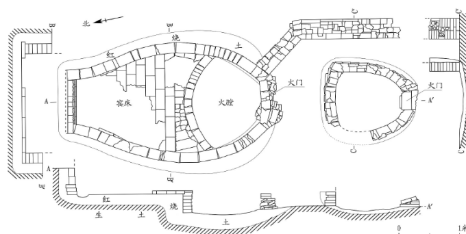
图五// Y1平、剖面图
