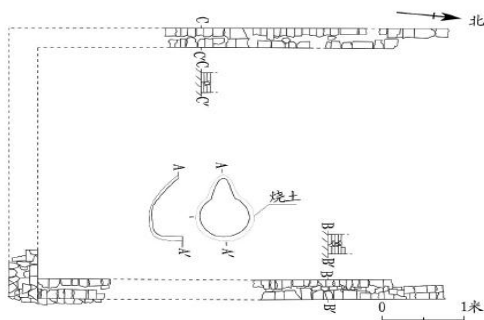
图七// F4平、剖面图
