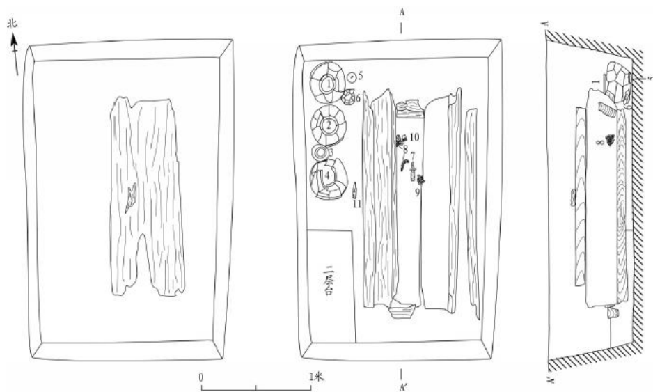
图九// M7平、剖面图
