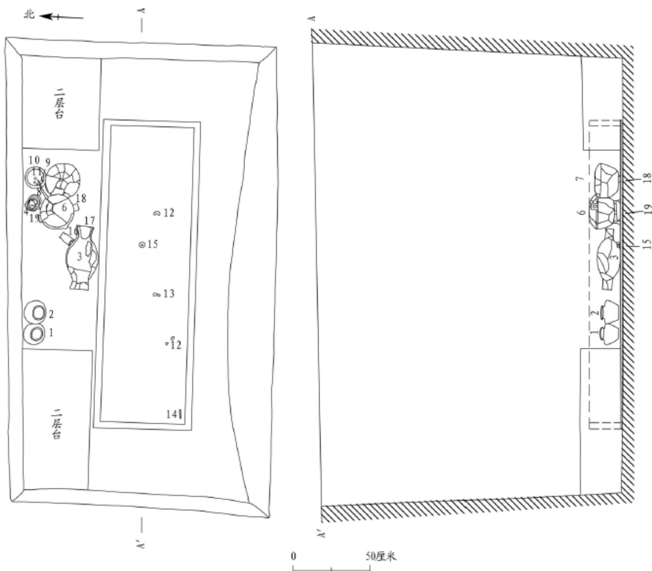
图四// M2平、剖面图
