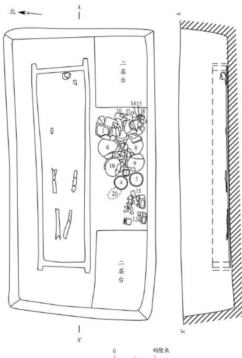
图八// M6平、剖面图
