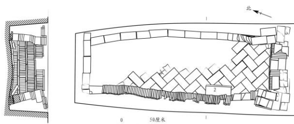
图五 M19 平、剖面图
