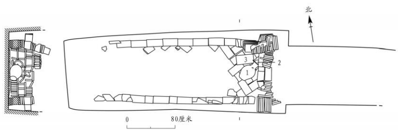
图二//M15 平、剖面图
