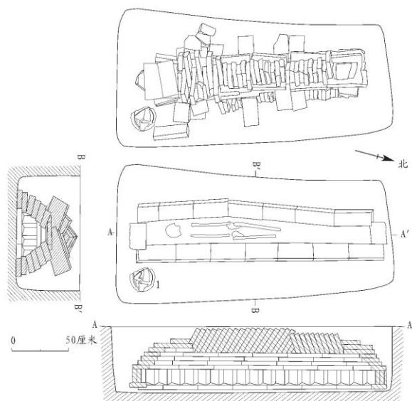
图一四//M15 顶面、平面、剖视图
