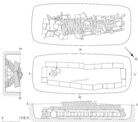
图一三//M10 顶面、平面、剖视图
