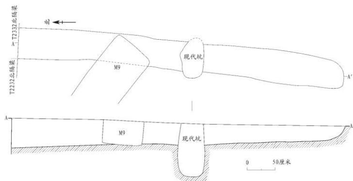
图一八//G1 平、剖面图
