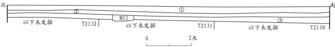
图三//T2130、T2131、T2132 东壁图
