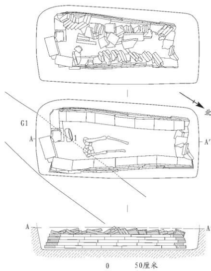
图一二//M9 顶面、平面、剖视图
