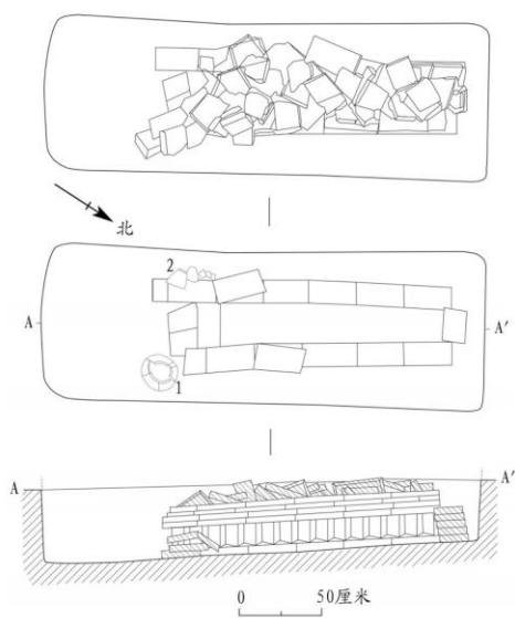
图八//M1 顶面、平面、剖视图
