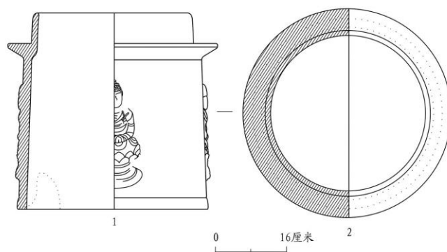
图二一塔刹铁套筒（东阳）
