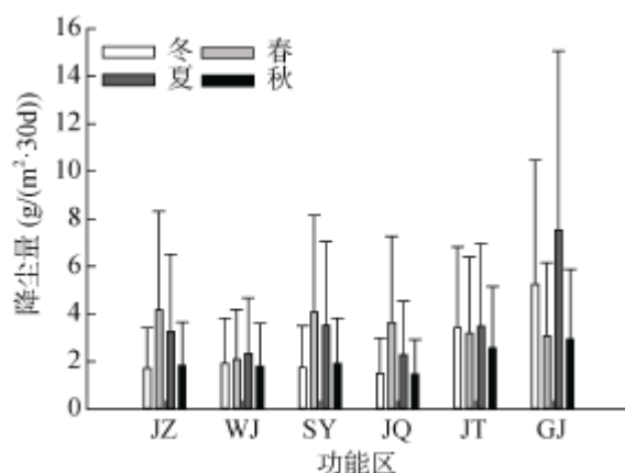
图 1 不同功能区各季节降尘通量的变化趋势
