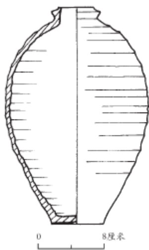
图六//陶瓶 (M1:7)
