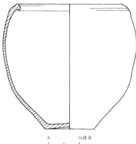
图五//陶油缸 (M1:1)
