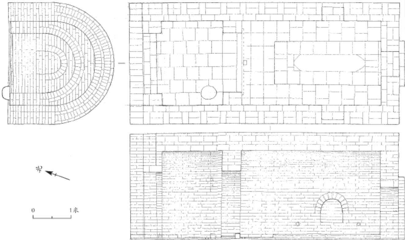
图二//杨庆墓(05NJZM1)平、剖面图
