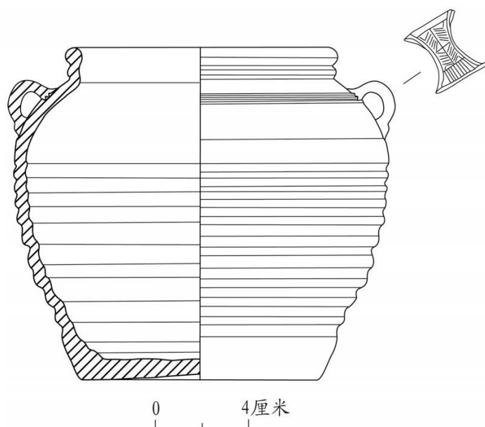
图五//M24 出土釉陶罐 (M24:2)
