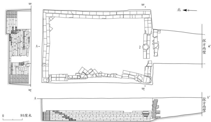
图三//M24 平、剖面图
