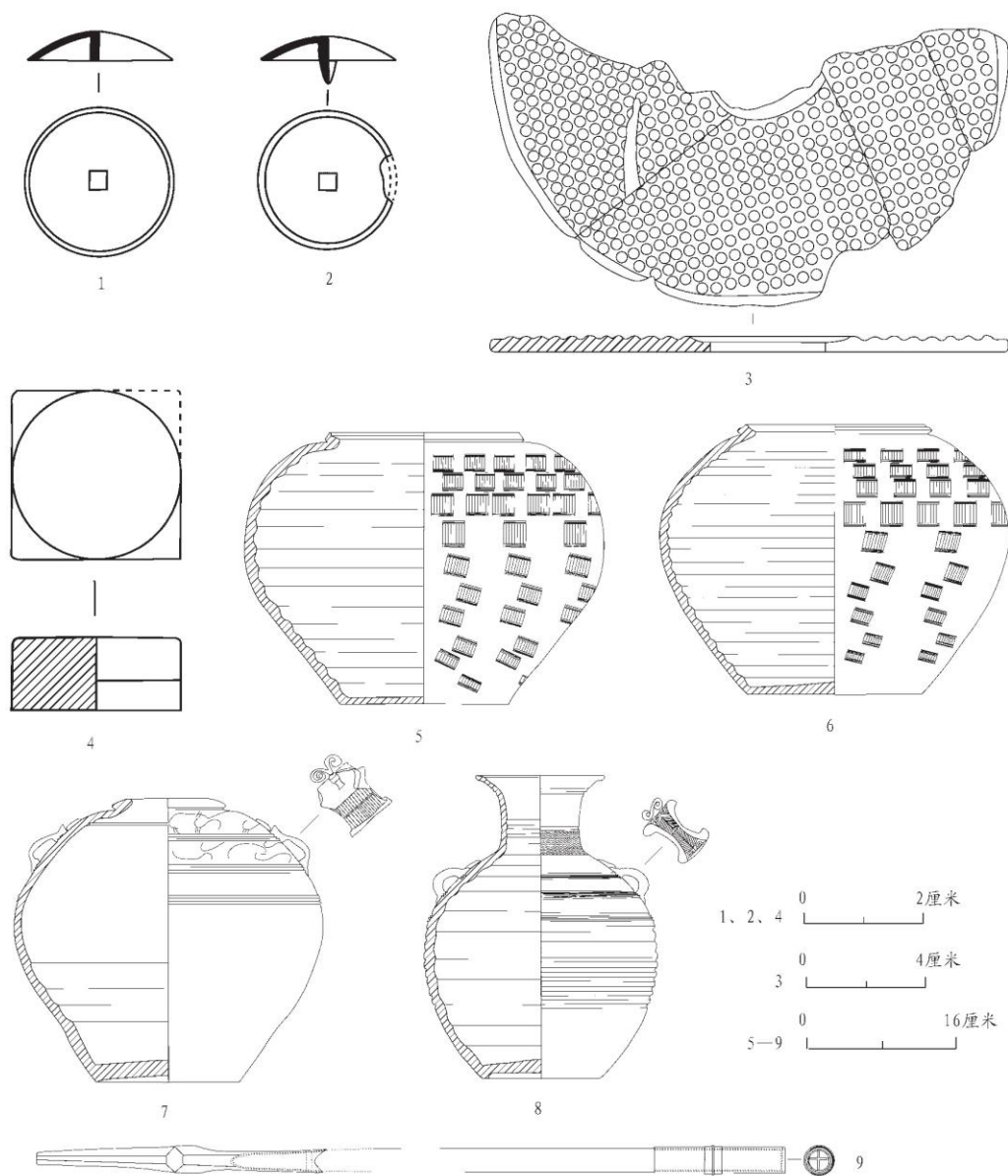
图一五//M44 出土器物
