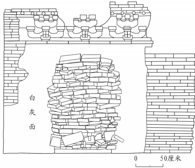
图三//M1 封门图
