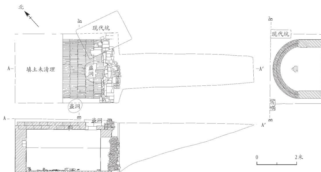
图二//M1 顶部平、剖面图
