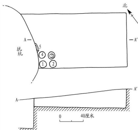
图六 D2M2 平、剖面图
