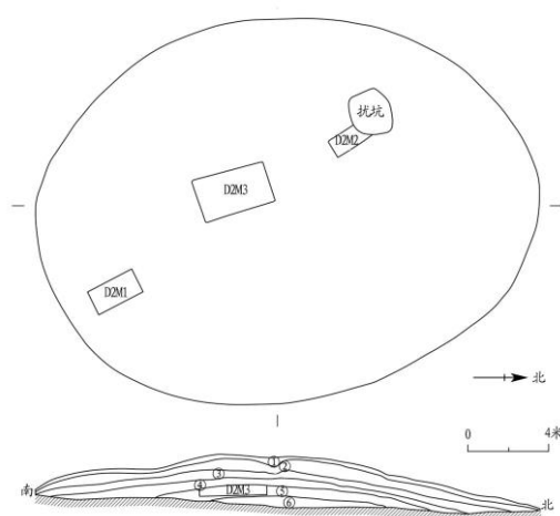
图二 D2 平、剖面图
