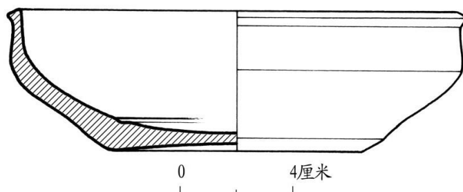
图三 硬陶碗（D2(3)：1）
