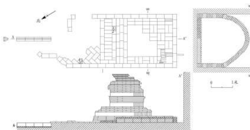
图二//M1 平、剖面图
