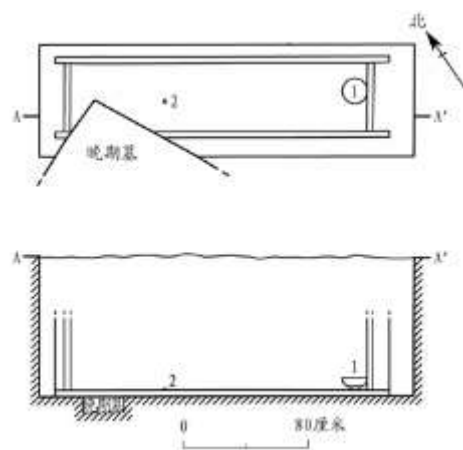
图八//M15 平、剖面图
