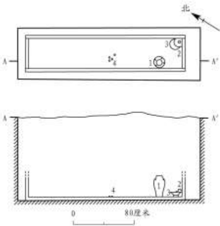
图一七//M28 平面图
