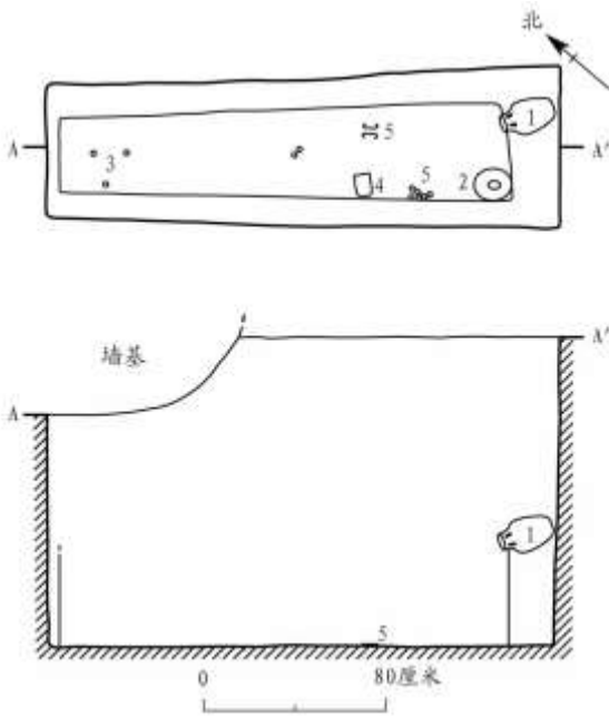
图四//M3 平、剖面图
