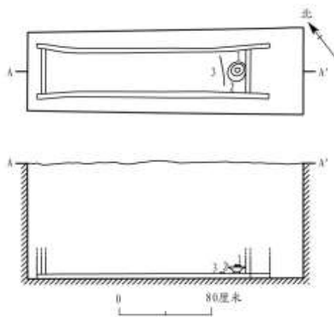
图一二//M20 平、剖面图
