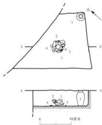
图二二//M50 墓葬平、剖面图
