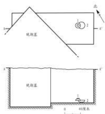
图七//M13 平、剖面图
