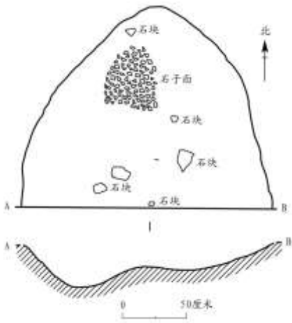
图一三//H5 平、剖面图
