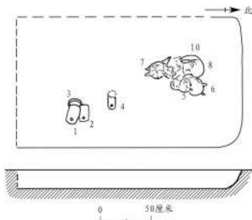
图一〇//M22 平、剖面图
