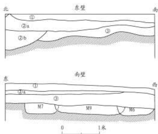
图七//T0814 东壁、南壁剖面图
