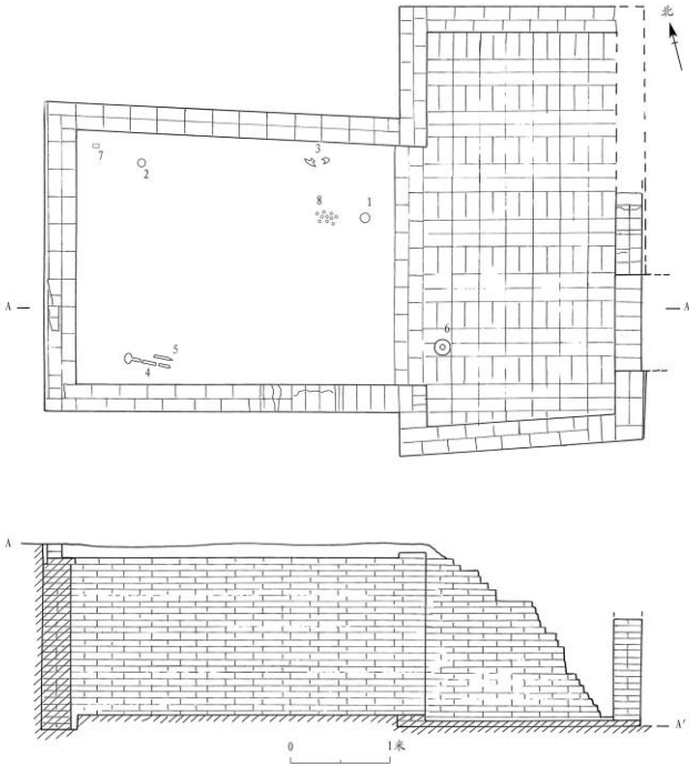
图二//M1 平、剖面图
