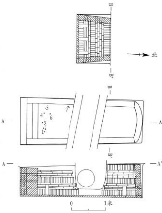
图三//M1 平、剖面图
