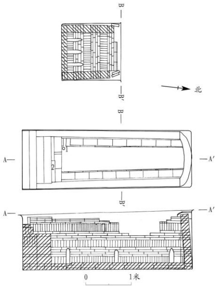
图八//M3 平、剖面图
