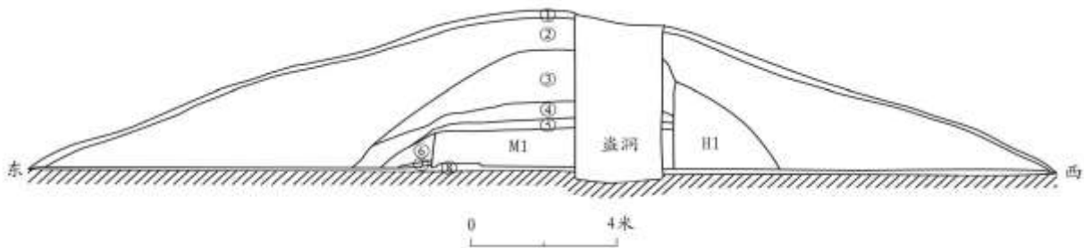
图二//D1T1、T2 南壁剖面图
