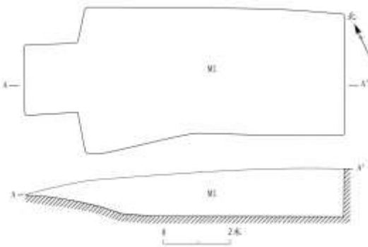
图一〇//D2M1 平、剖面图
