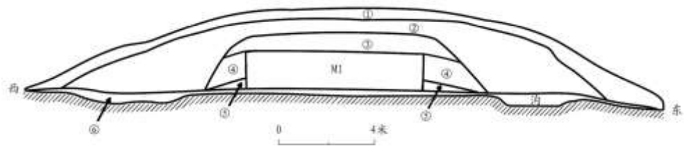
图七//D2T3、T4 北壁剖面图
