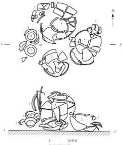
图九//D2Q1 平、剖面图
