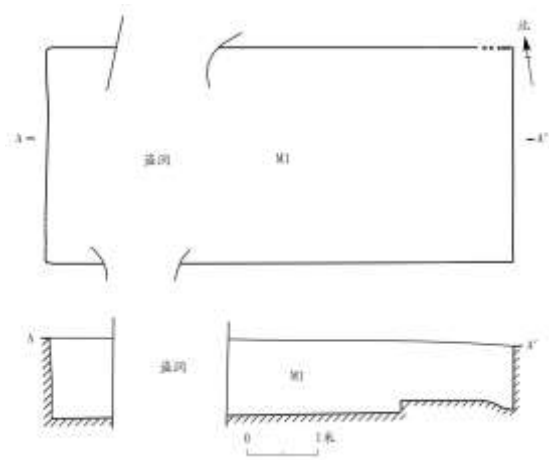
图五//D1M1 平、剖面图
