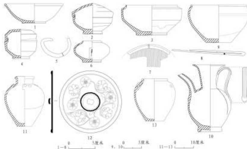
图七// II M29 出土器物
