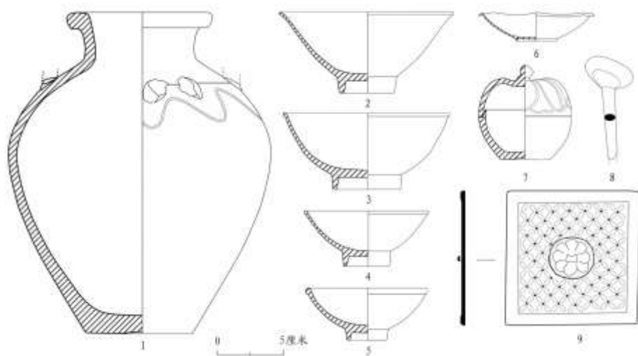
图一九//IM41 出土器物
