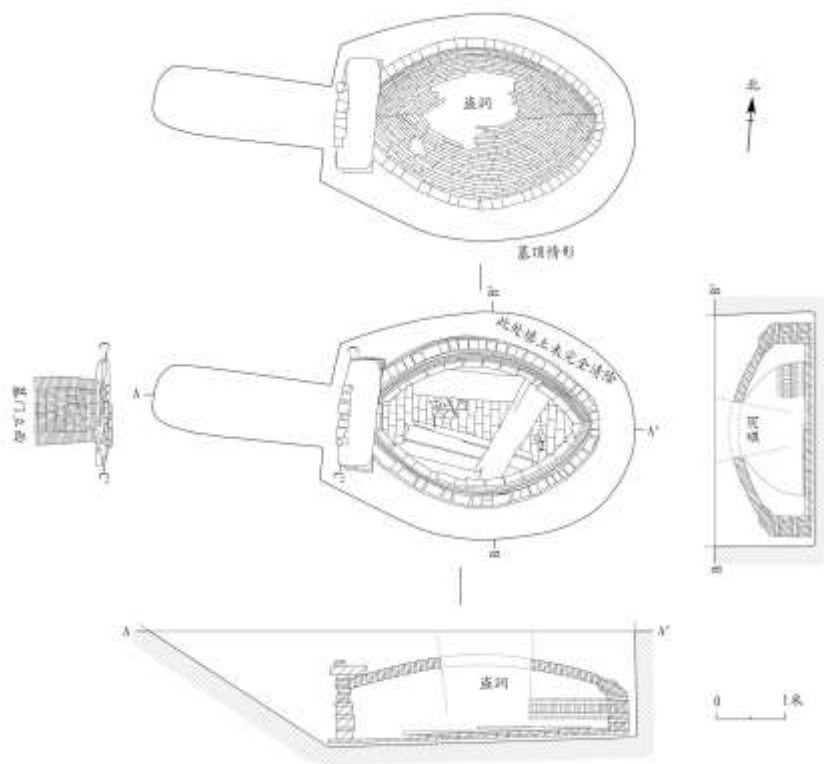
图一四//II M30 顶面、平面、剖视图、墓门立面图 1. 瓷壶
