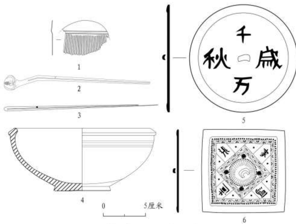
图一七// II M31 出土器物
