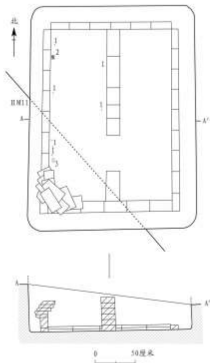
图五// II M4 平面、剖视图 1. 棺钉 2. 铜钱 3. 铁环
