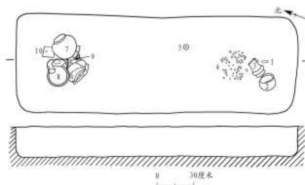
图六//M13 平、剖面图 3. 4. 5. 6.
