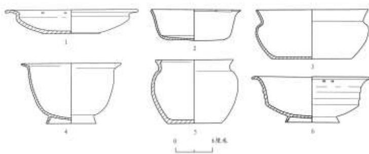
图一一//出土陶盆、圈足盘
