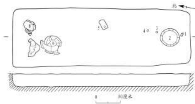
图五//M5 平、剖面图
