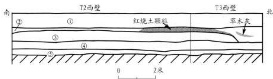
图四//朱家兜遗址 T2、T3 西壁地层剖面图
