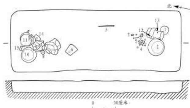
图七//M19 平、剖面
