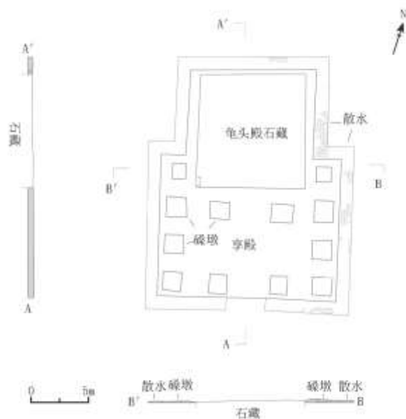
图五享殿与龟头殿基址平剖面图
