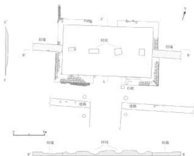
图七门殿基址平、剖面图
