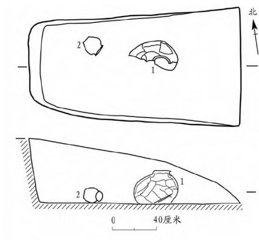
图九//D1M2 平、剖面图
