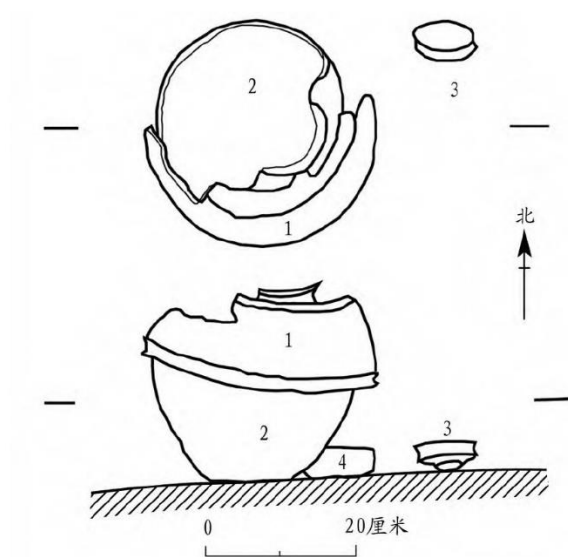
图一八//D1Q4 平面图
