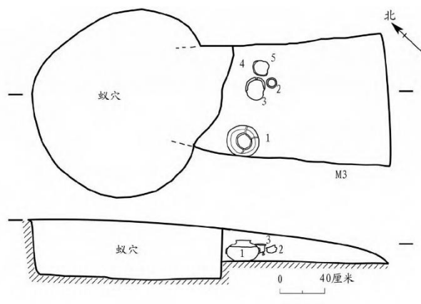
图一〇//D1M3 平、剖面图
