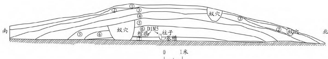
图三//杨家山 D1 南北向隔梁东侧剖面
