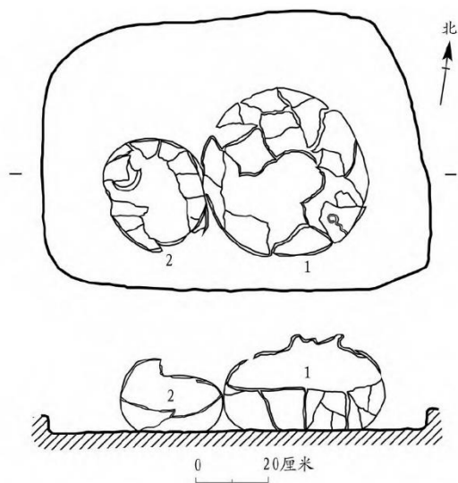
图一九//D1Q5 平、剖面图
