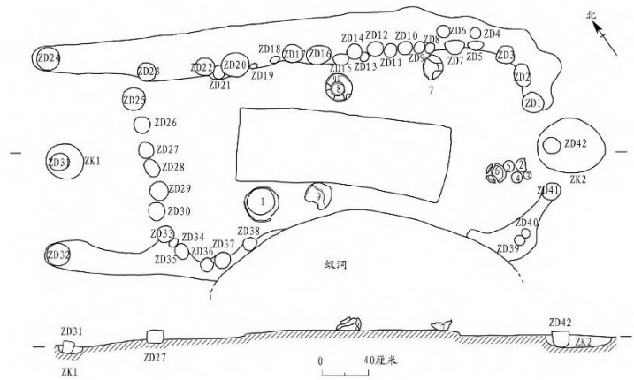
图一三//D1M5 平、剖面图
