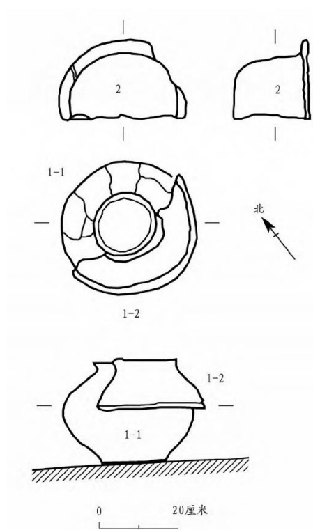
图一七//D1Q3 平、剖面图
