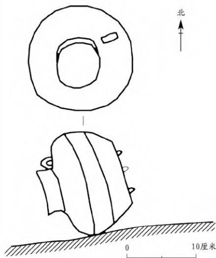
图二二//D1Q8 平、剖、侧面图
