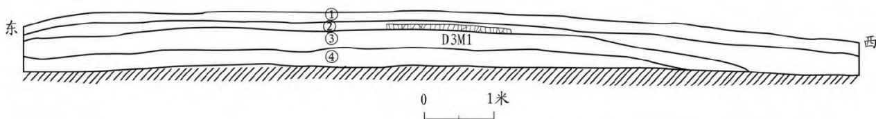
图四//杨家山 D3 东西向隔梁北侧剖面
