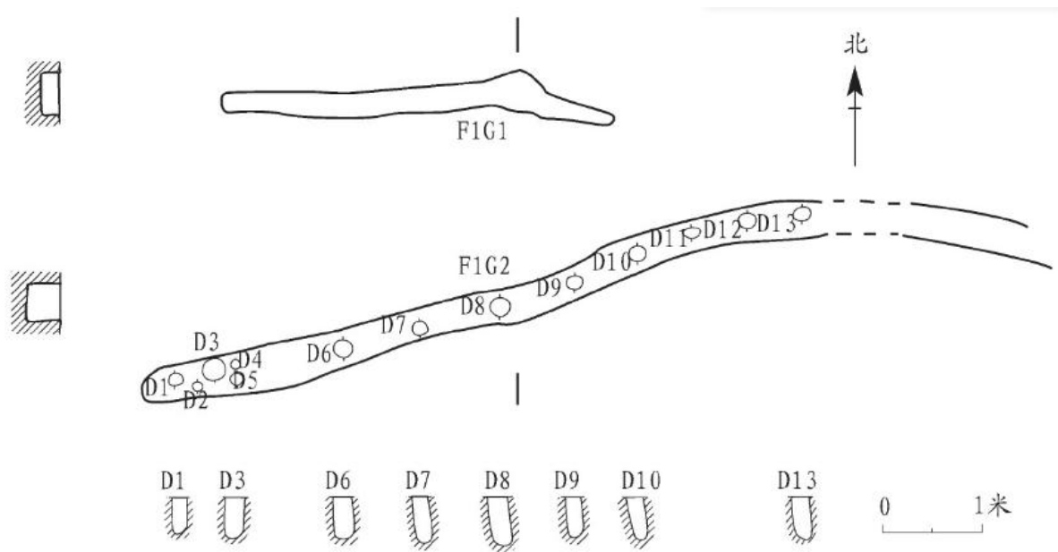
图一五//D1F1 平、剖面图
