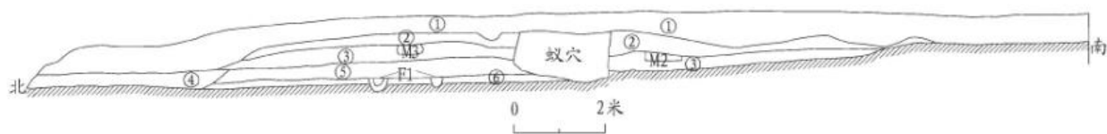
图一六//D2T2、T3 东壁地层图
