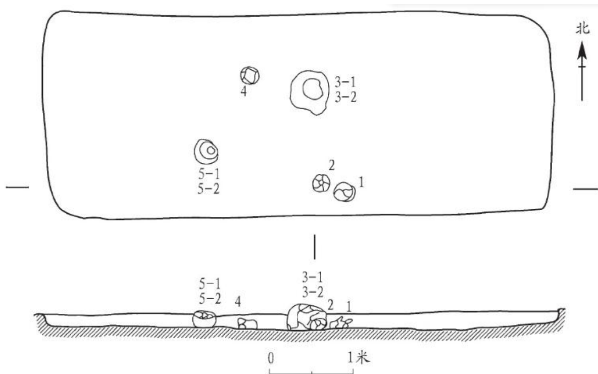
图一〇//D1M6 平、剖面图
