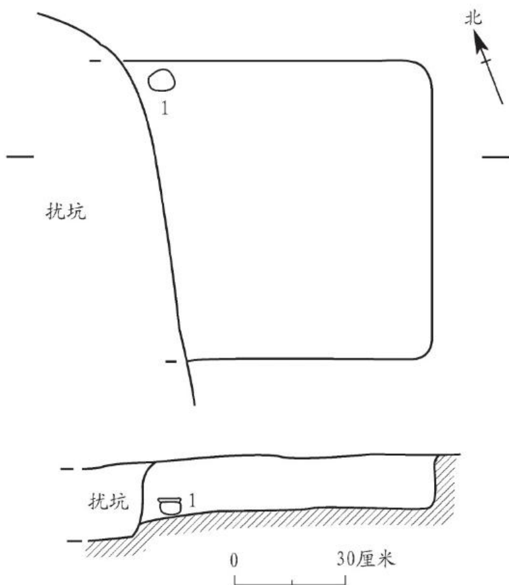
图一八//D2M1 平、剖面图
