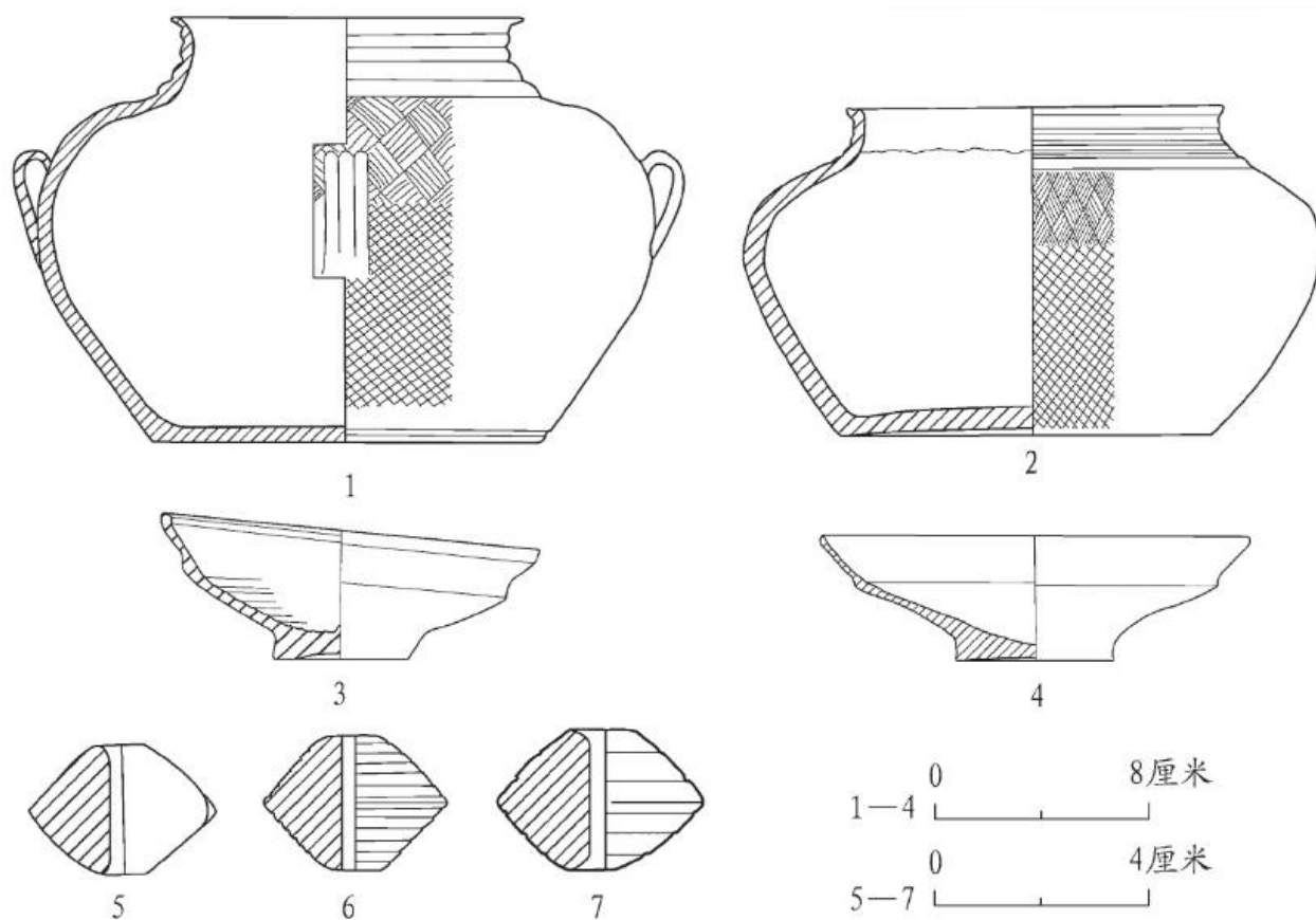
图二五//D2Q1 出土器物
