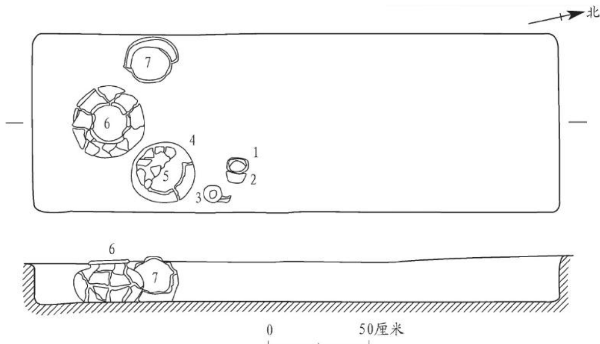
图四//D1M1 平、剖面图
