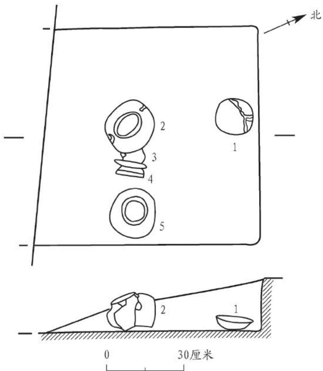
图一九//D2M2 平、剖面图
