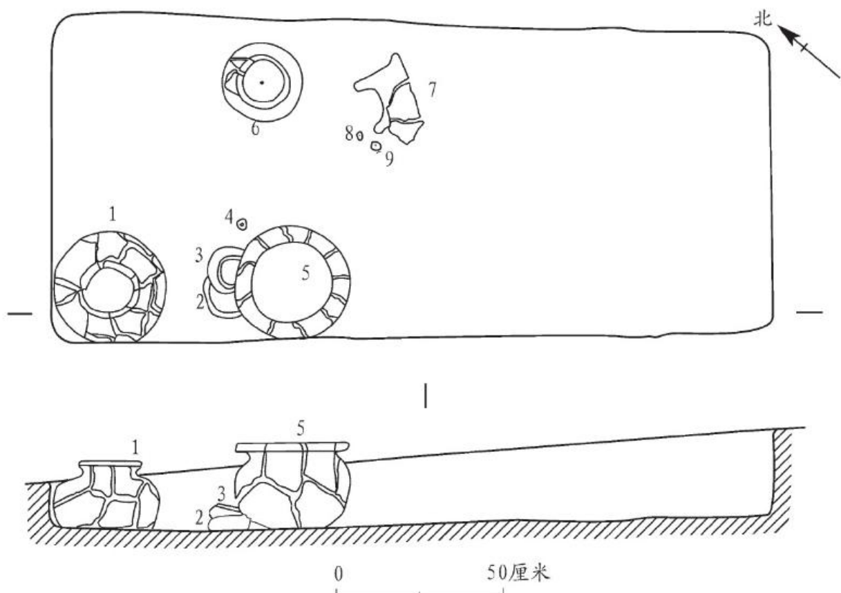
图八//D1M5 平、剖面图
