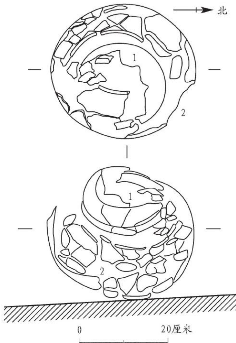
图一二//D1Q1 平、剖面图
