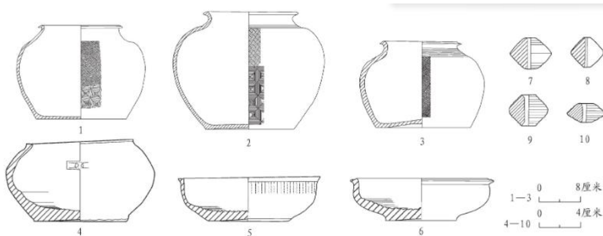
图九//D1M4、D1M5 出土器物
