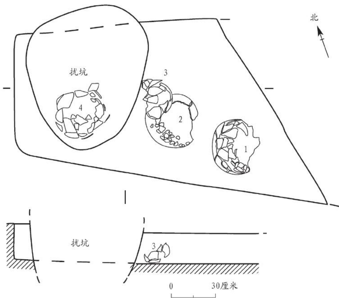
图六 D1M2 平、剖面图
