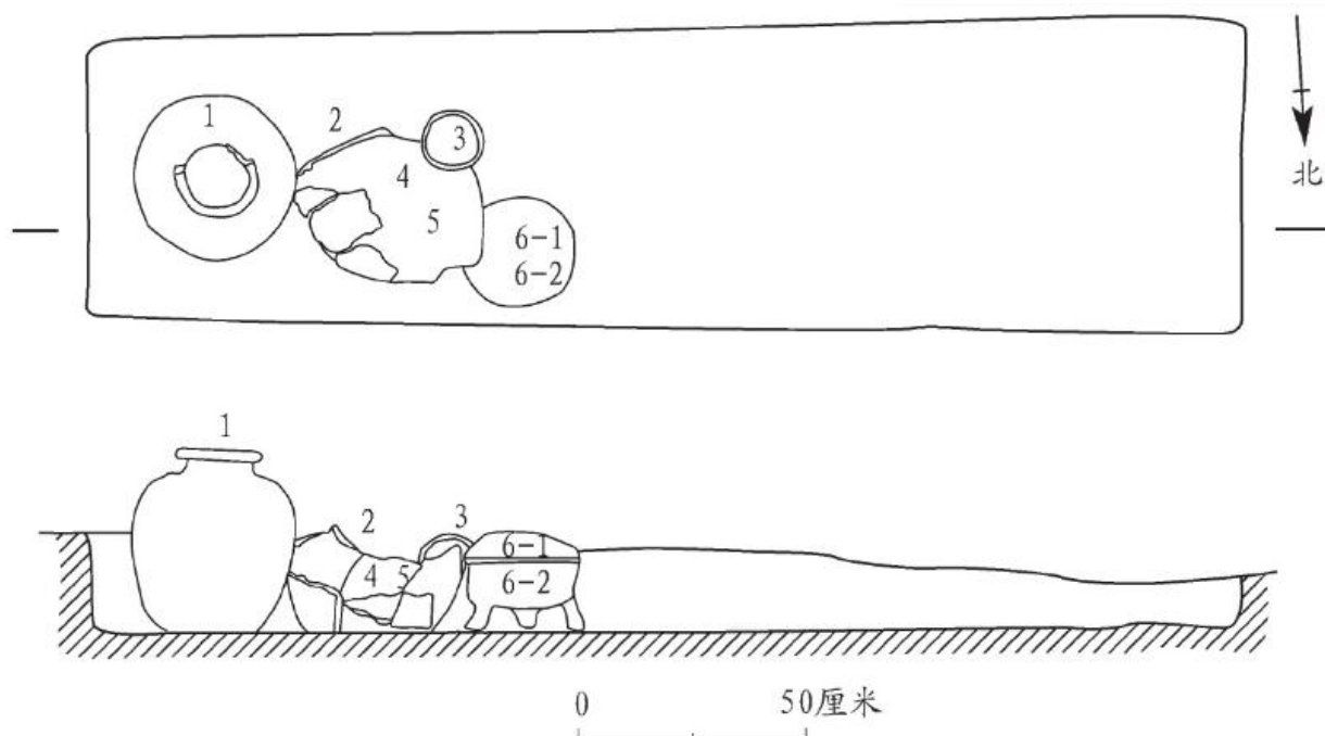
图二一//D2M3 平、剖面图
