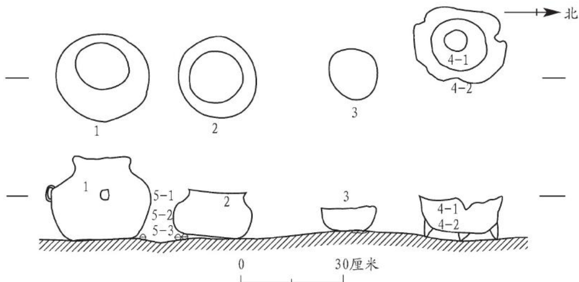
图二四//D2Q1 平、剖面图
