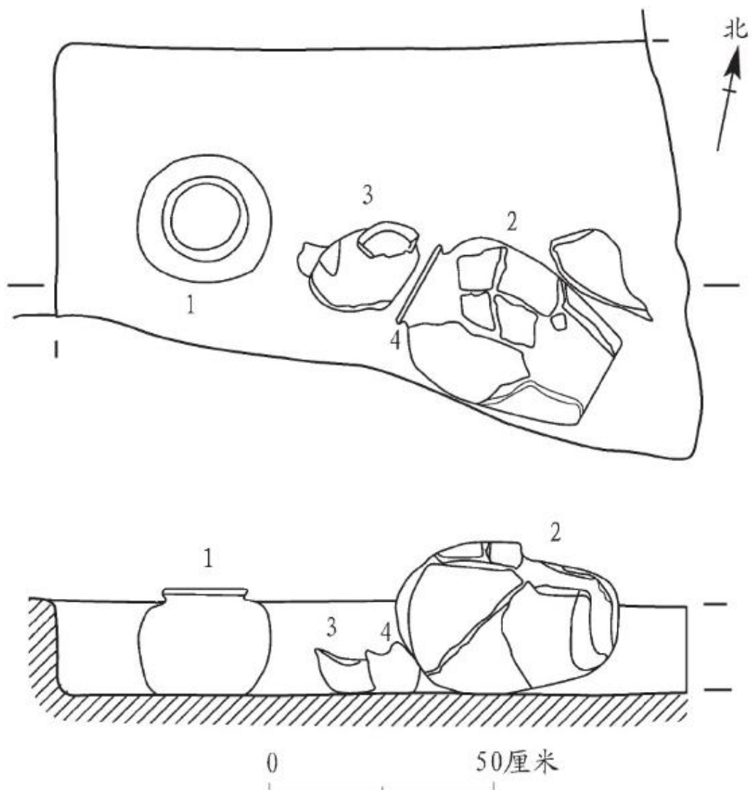
图二三//D2M4 平、剖面图
