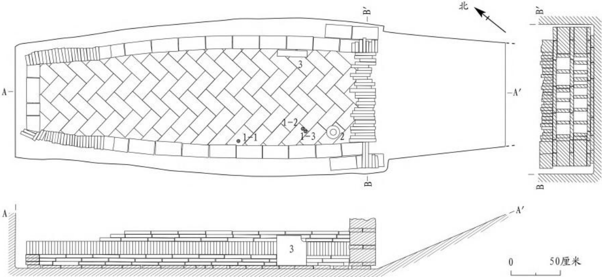
图四// M15平、剖面图 1.铜钱 2.青瓷钵 3.砖质墓志
