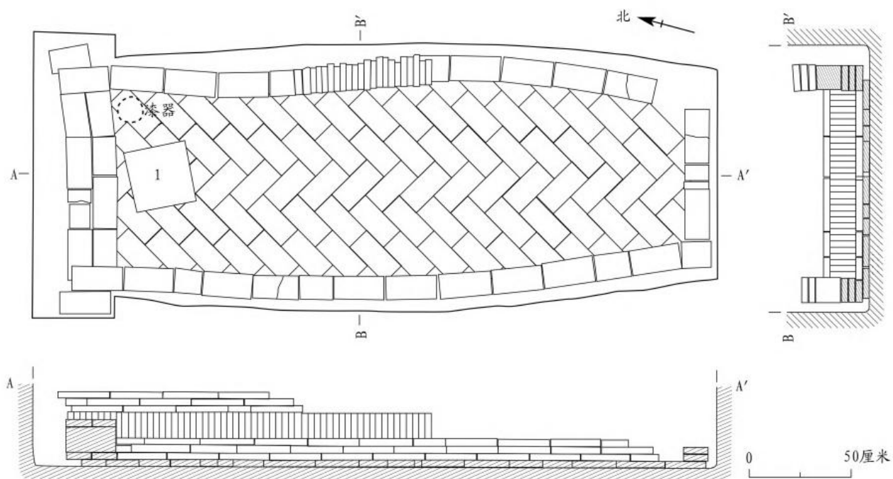
图二// M10平、剖面图
