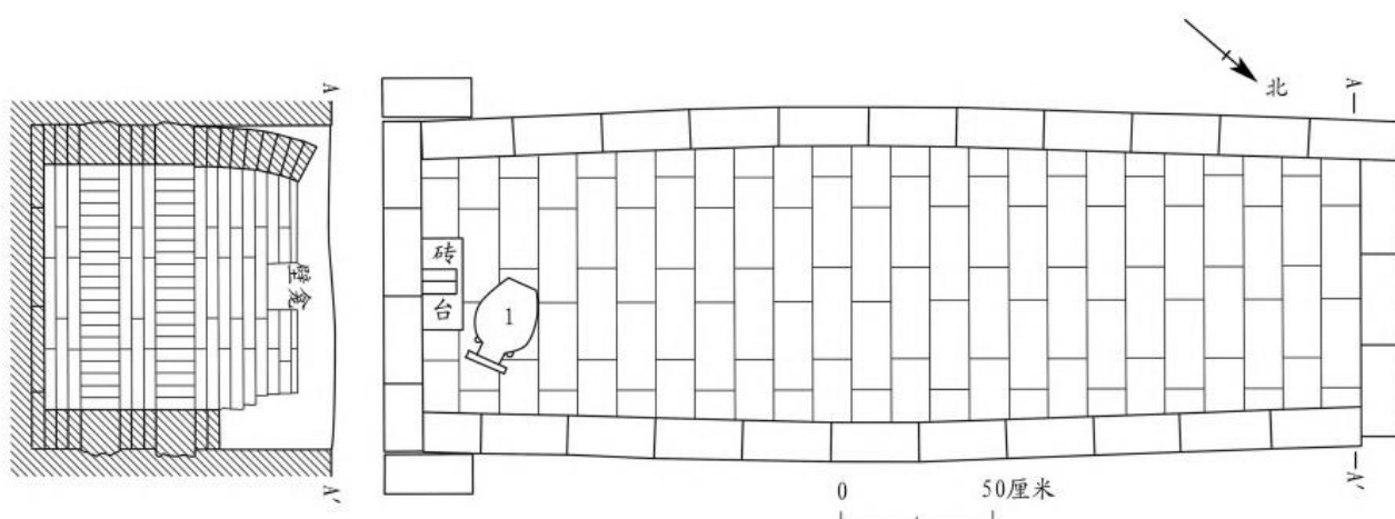
图一四// M42 平、剖面图
