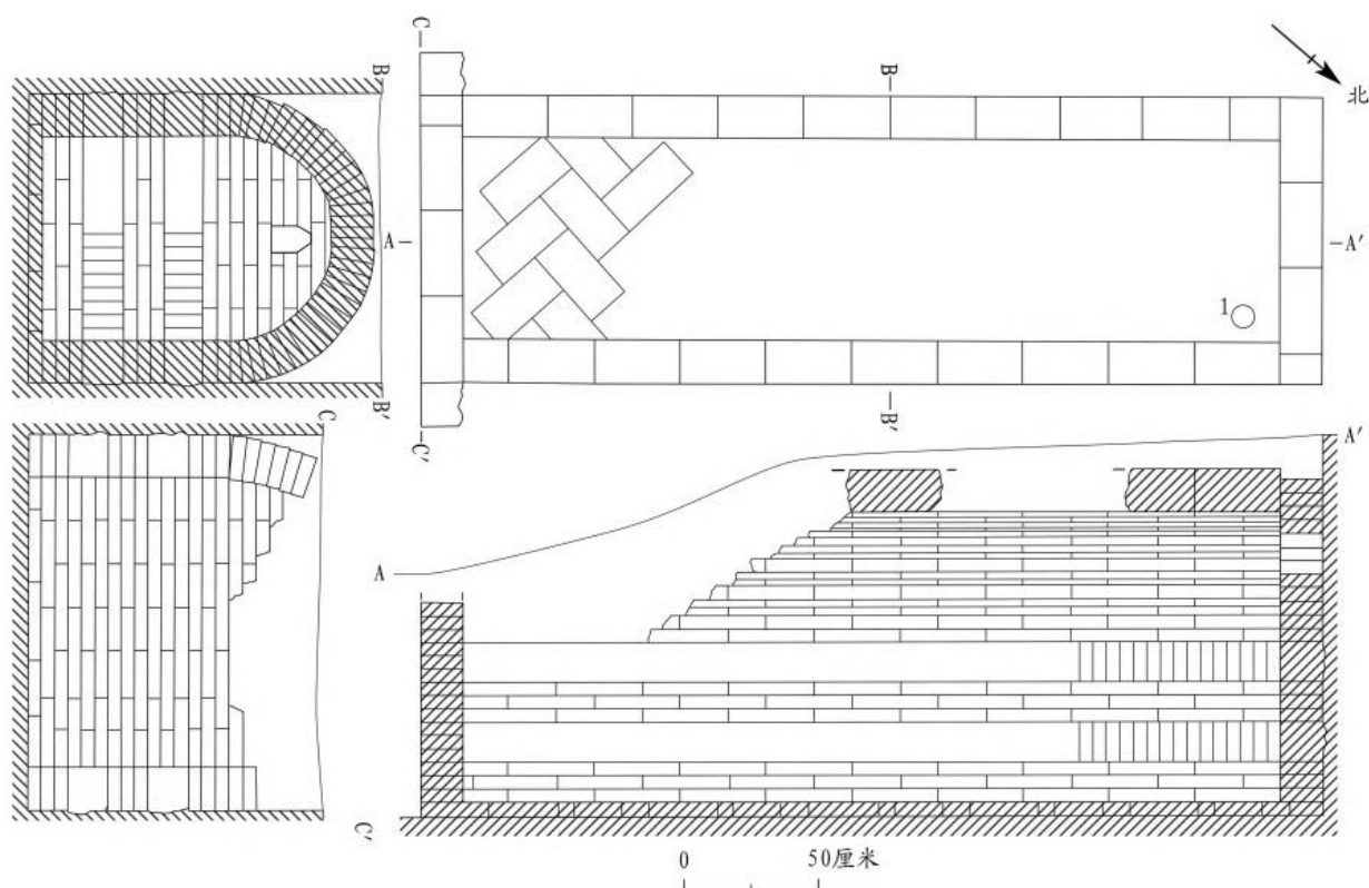
图五// M10平、剖面图
