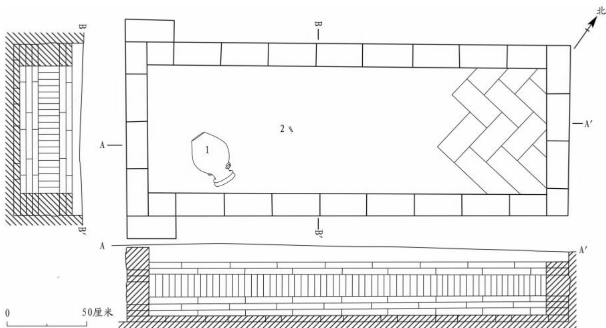
图一三// M27 平、剖面图
