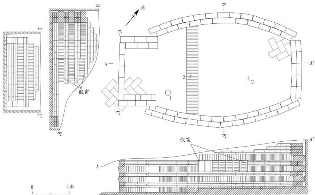
图七// M12平面、剖视图
