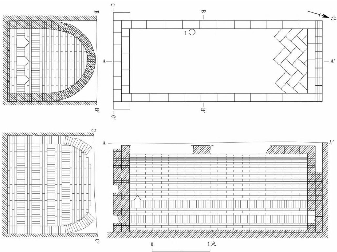
图三// M9平、剖面图
