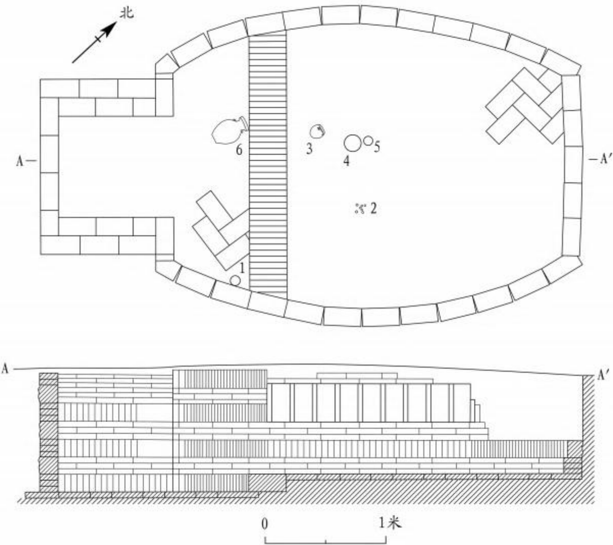
图一七// M54平面、剖视图
