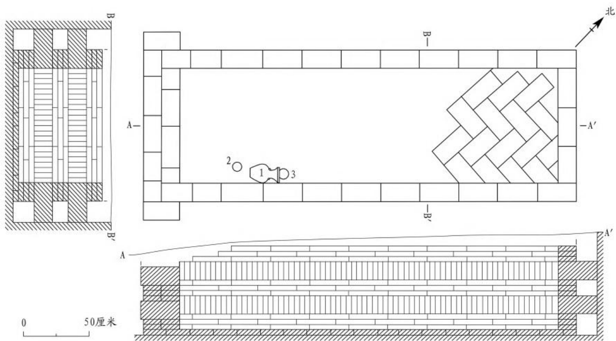
图一〇// M22平、剖面图
