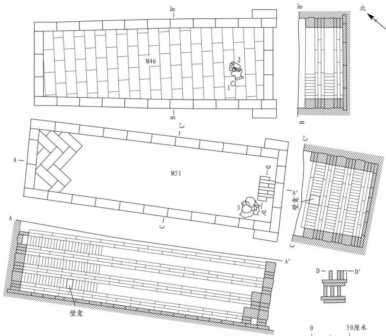
图一五// M46、M51平、剖面图 1.青瓷碗 2、3.青瓷盘口壶(M46:2、M51:1)
