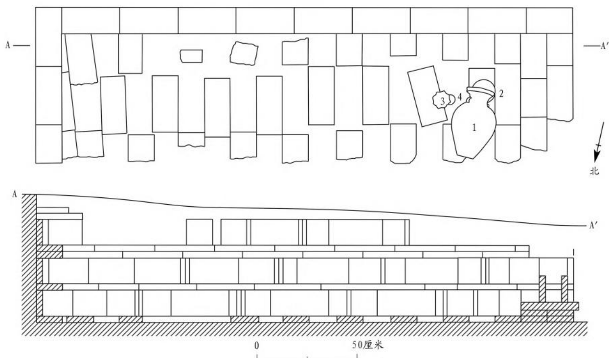
图一二// M23平、剖面图
