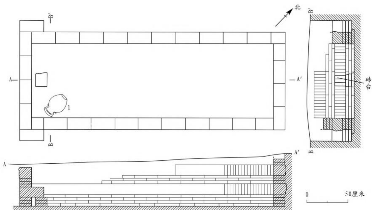
图一六// M53 平、剖面图
